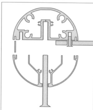
Schnittbild Entrée mit Abdeckprofil rund.
