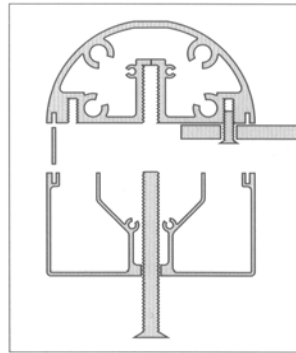
Schnittbild Entrée mit Abdeckprofil eckig.
